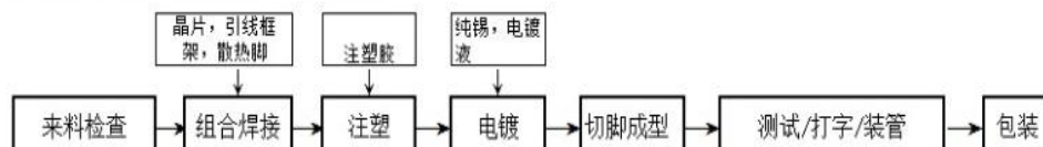
图 4.3-1 二极管、三极管生产工艺流程图
